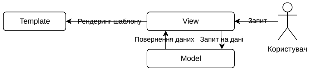
Рисунок 2.1 — Схема для фреймворку
